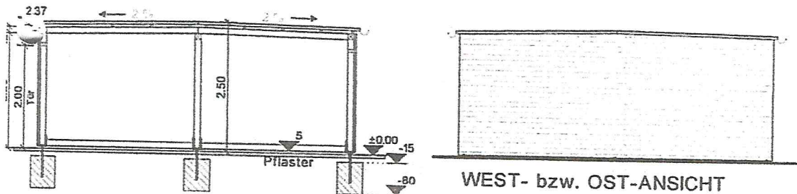
SCHNITT A-A
