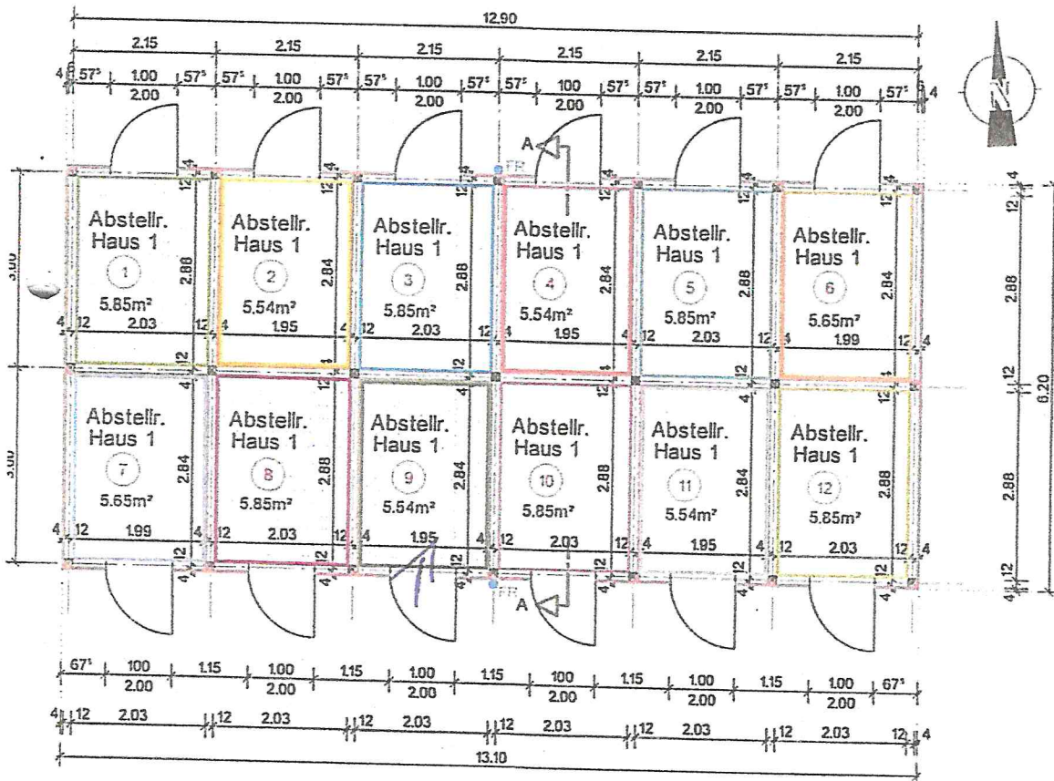
GRUNDRISS
