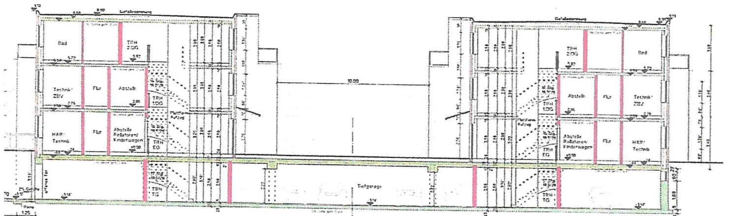
SCHNITT B-B (Gerzen) Haus 2
