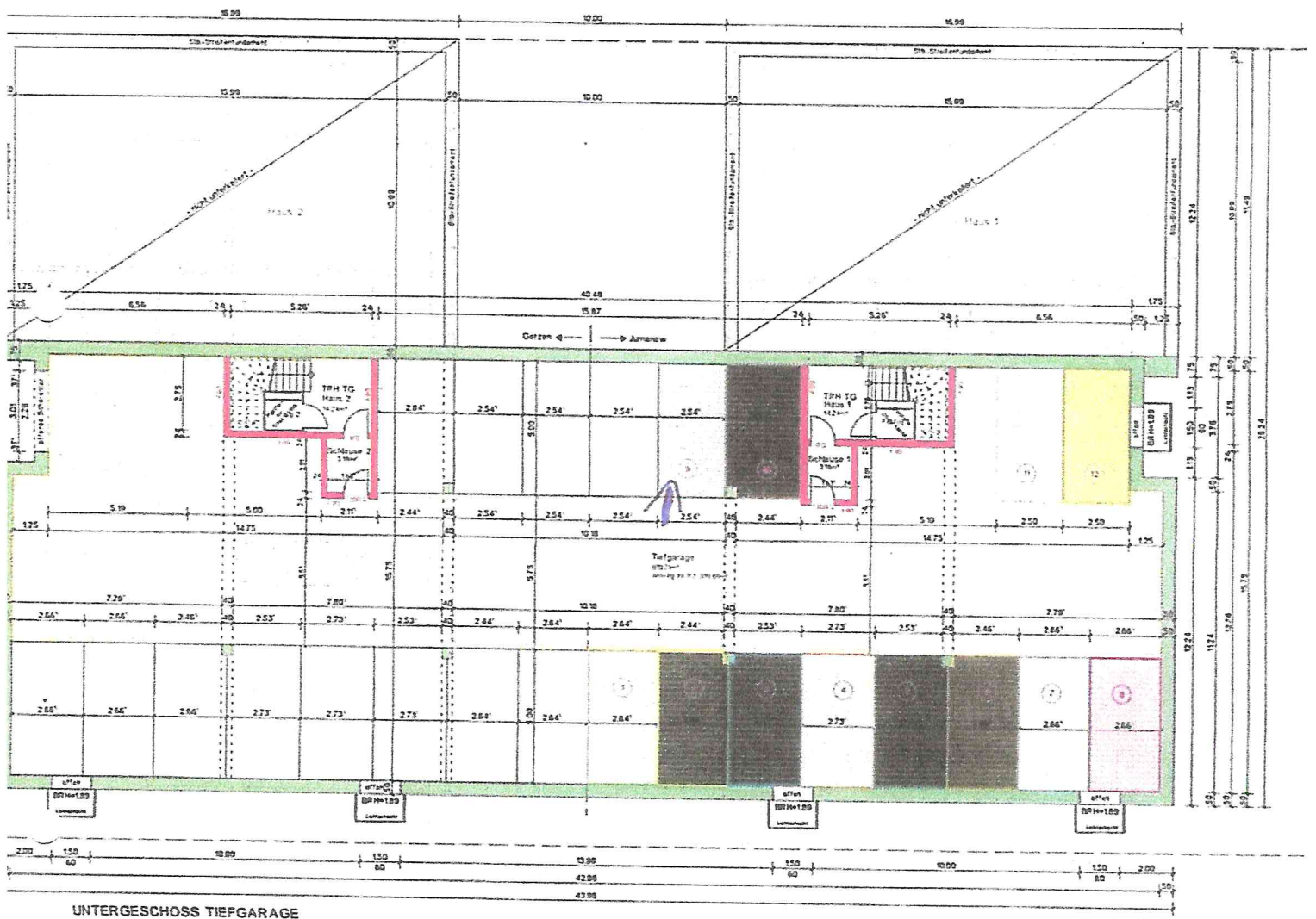
UNTERGESCHOSS TIEFGARAGE
